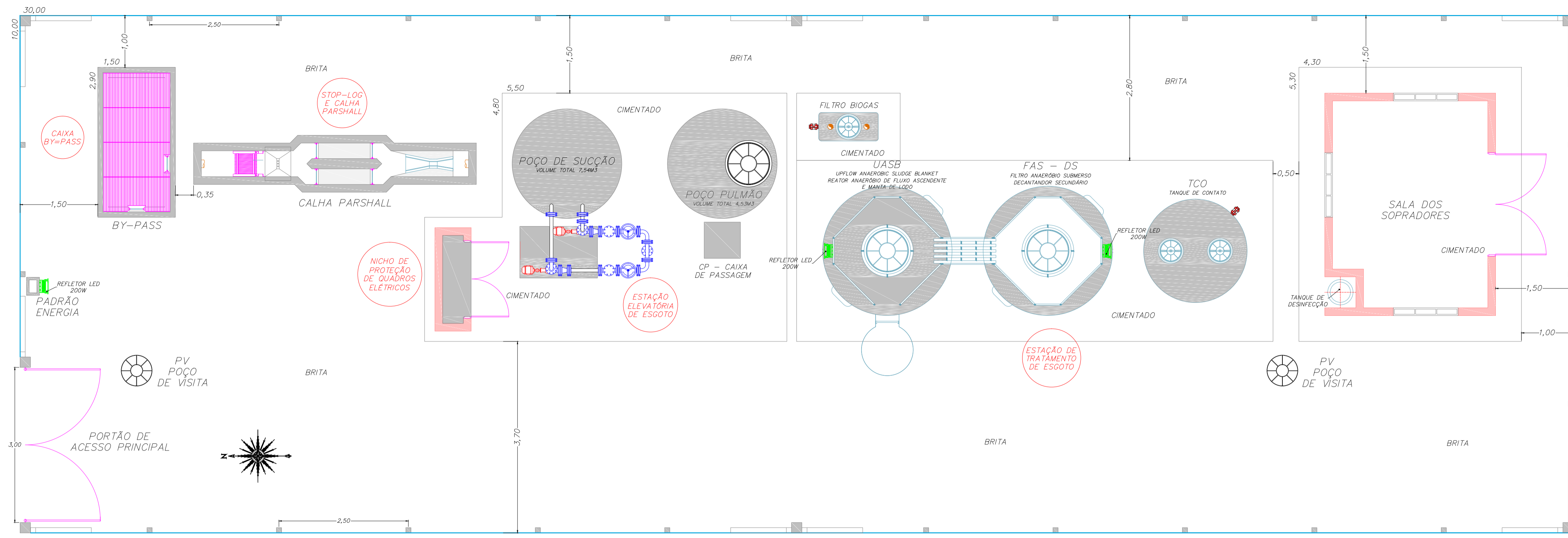
IMPLANTAÇÃO ESCALA 1:50
